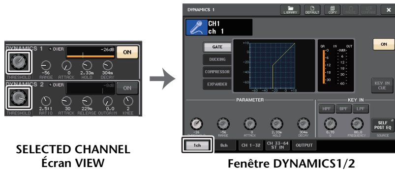
Fenêtre DYNAMICS1/2
